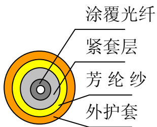
单芯室内光缆
