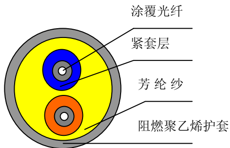
双芯室内光缆
